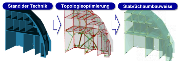
BILD 9. CFK-Stab/Schaum Verbundbauweise
