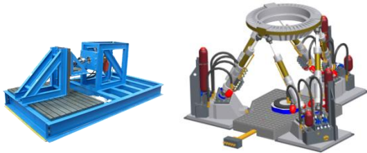
BILD 11. Hydropulser und Hexapodprüfanlage
