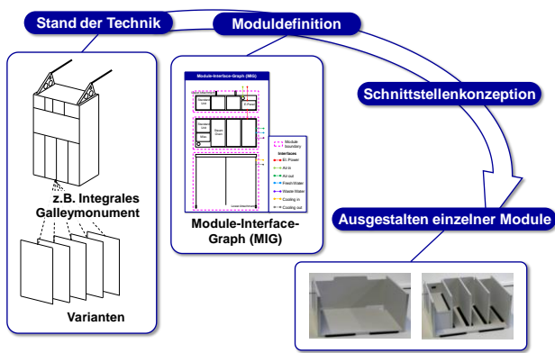
BILD 2. Entwicklung Modulkonzept
