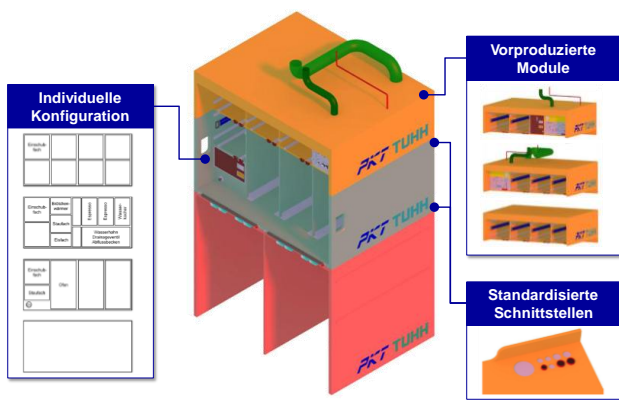
BILD 5. Konzept Widebody-Modulgalley
