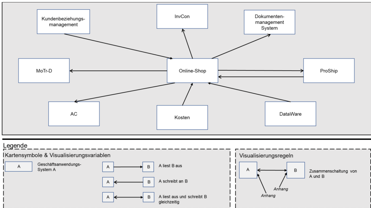
Abbildung 10: Softwarekarte ohne Verortung (Graphlayoutkarte) (eigene Darstellung nach Buckl et al. 2008)
