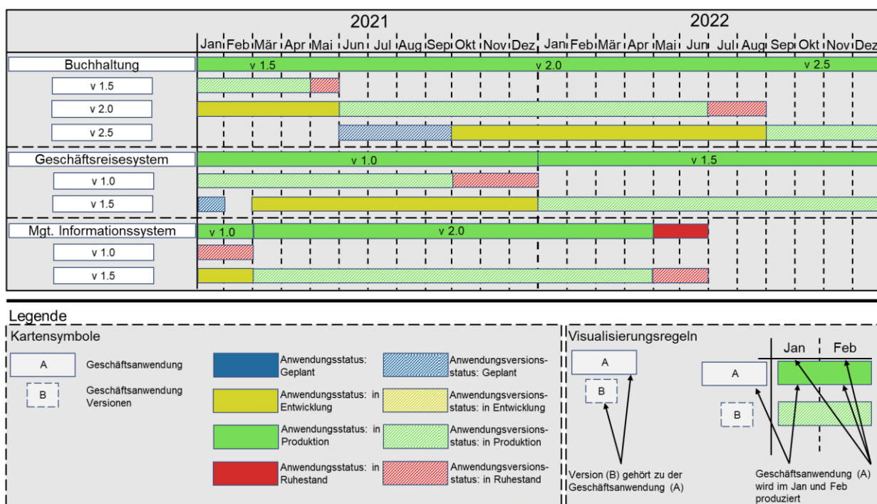
Abbildung 9: Zeitintervallkarte (eigene Darstellung nach Buckl et al. 2008)
