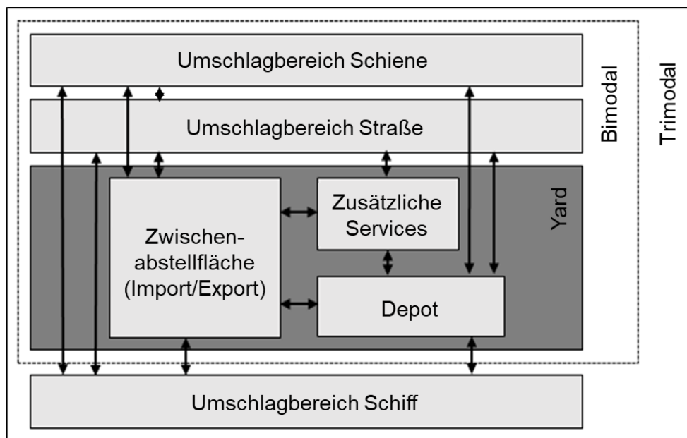
Abbildung 12: Funktionsbereiche innerhalb eines Binnen-Containerterminals (eigene Darstellung in Anlehnung an Böse 2007; Kaffka 2013)
