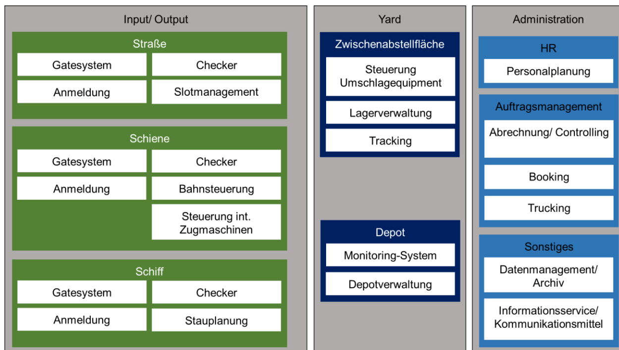
Abbildung 13: Generische Clusterkarte (Kartengrund) für Umschlagterminals (eigene Darstellung)
