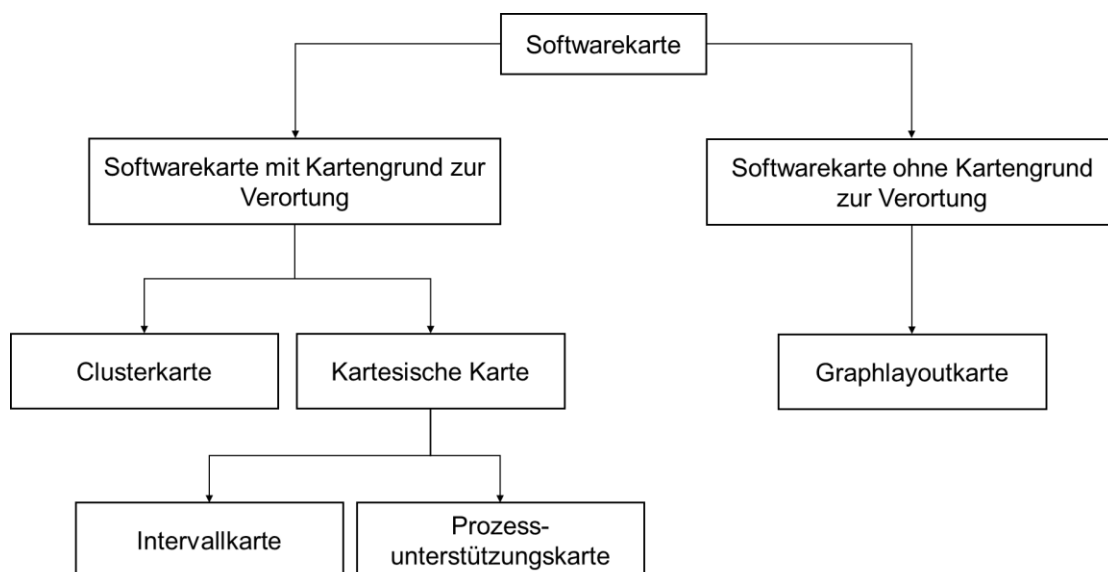
Abbildung 6: Vererbungshierarchie von Softwarekartentypen (eigene Darstellung nach Wittenburg 2007)
