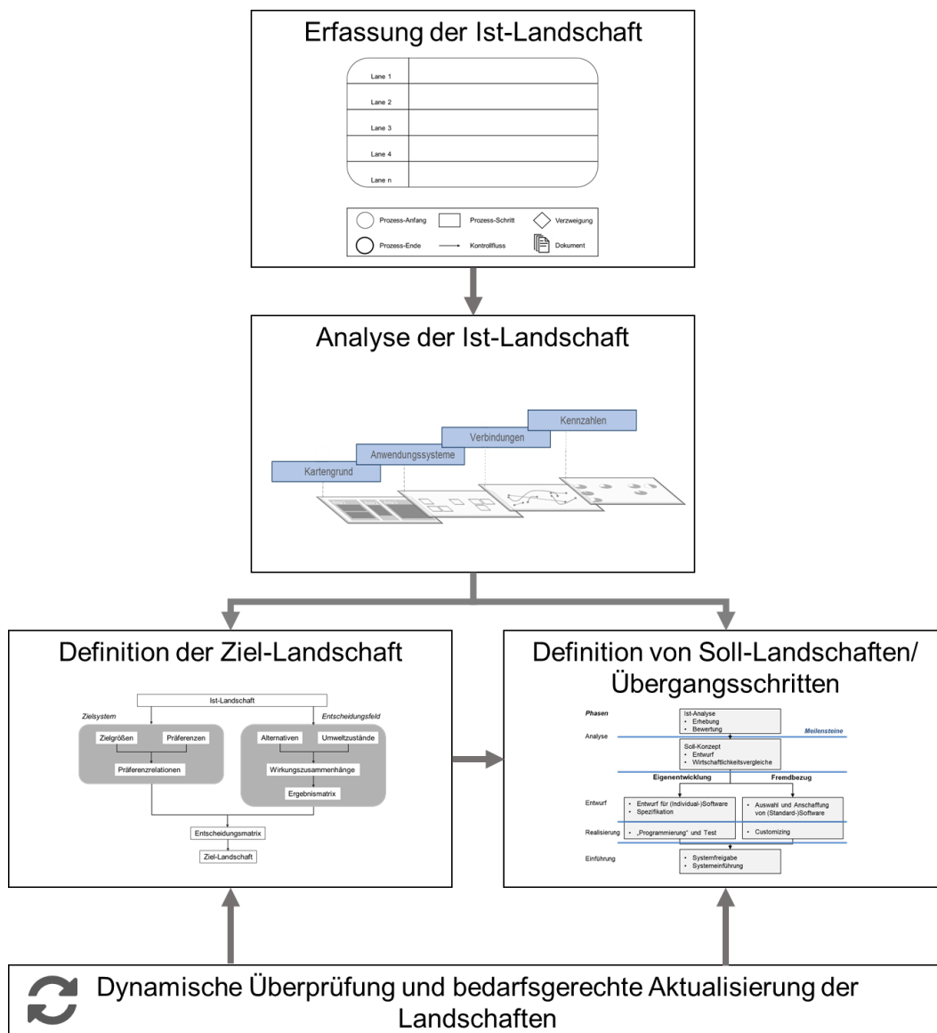
Abbildung 19: Zusammenwirken der einzelnen Vorgehensmodelle der Arbeitspakete in einem integrierten Referenzprozessmodell (eigene Darstellung)
